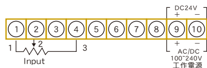
3 線電位計
