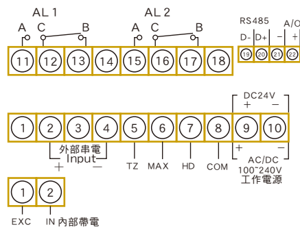
電壓/電流
