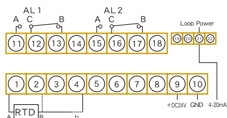
溫度(RTD)
