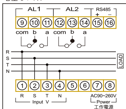
電壓 3Φ4W
