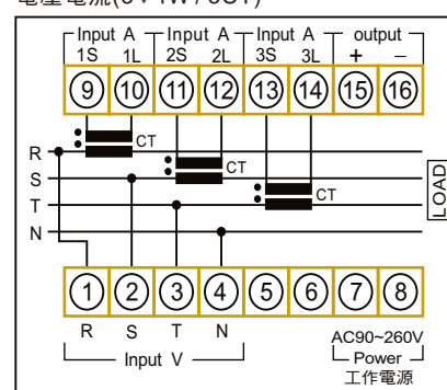
電壓電流(3Φ4W / 3CT)
